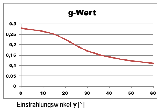
Abb. 2: g-Wert nach DIN EN 410 von OKAWOOD im 2-fach-Aufbau mit Wärmeschutzschicht
