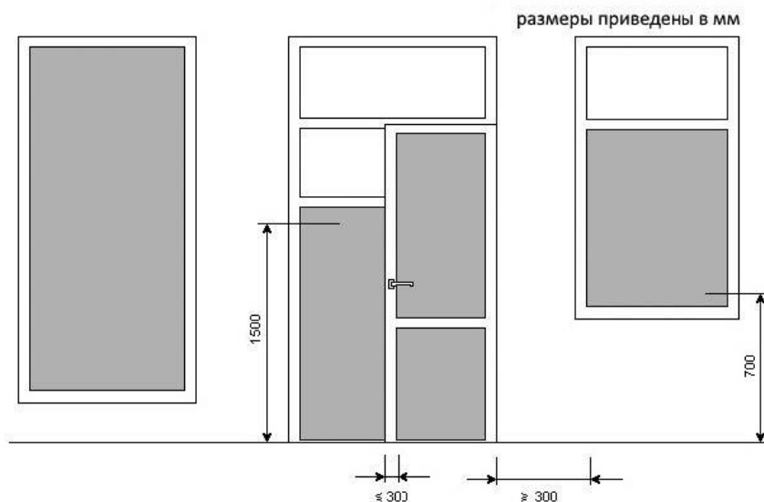
Рисунок 1: Применение безопасного ламинированного стекла VSG, VG
