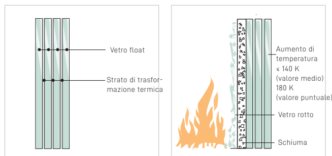
Struttura schematica di una vetrata antincendio EI
